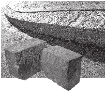
Bordures clivées, taillées grossièrement
