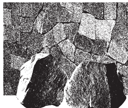
Pierres brutes de formes naturelles pour maçonnerie cyclopeenne
